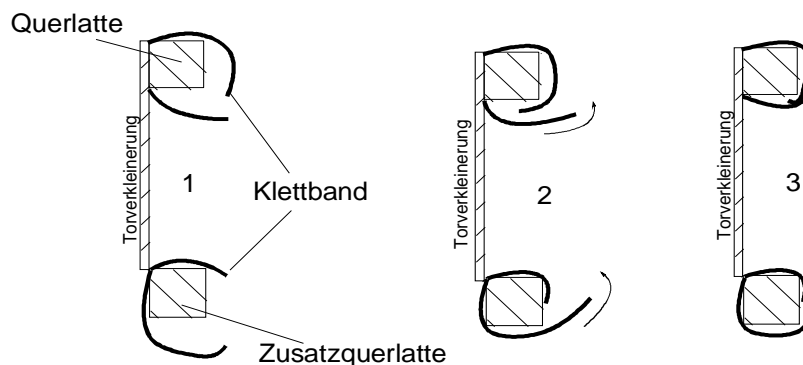
Abb. 2. Montage Torverkleinerung
