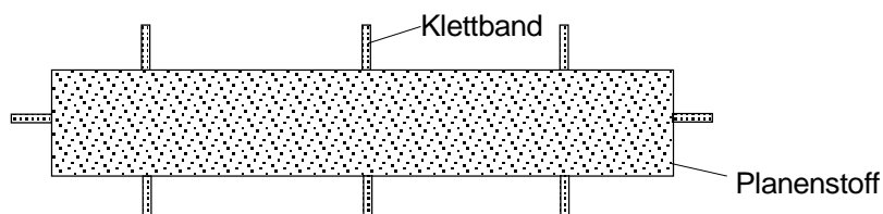
Abb. 2. Torverkleinerung
