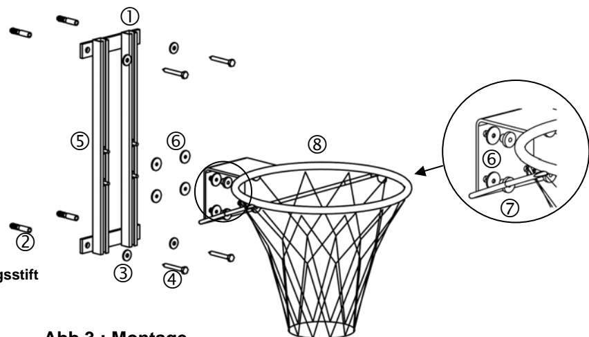
Abb.3 : Montage
