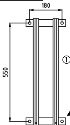
Abb. 2 : Bohrzeichnung
