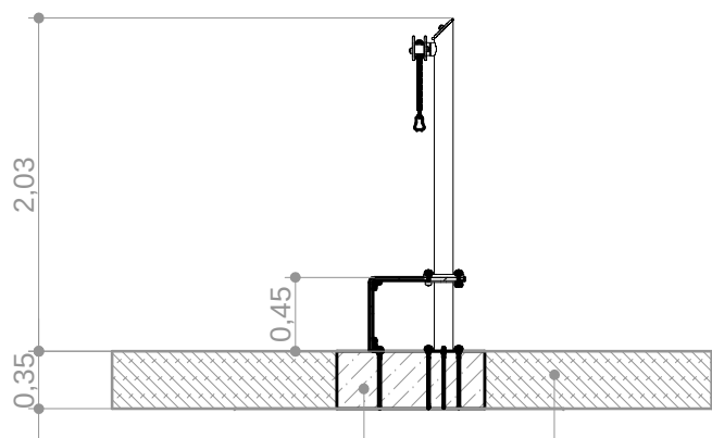
CORTE / SECTION A-A
