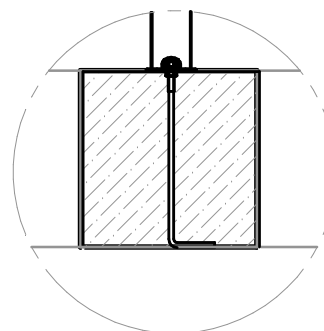
DETALLE ANCLAJE
