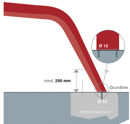
Bild 4 | Ausstiegsteil Verschraubung
