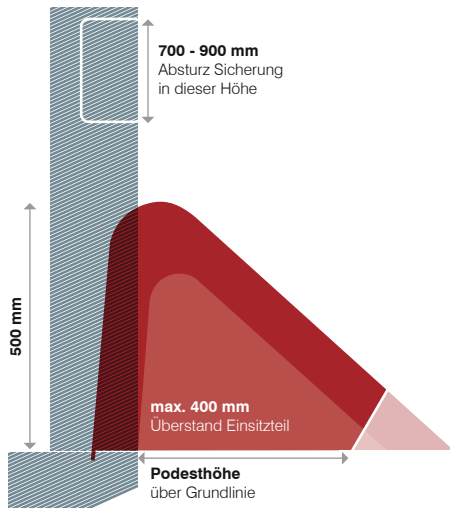
Bild 1 | Einstiegsteil
