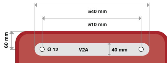
Bild 2 | Einstiegsteil Befestigung
