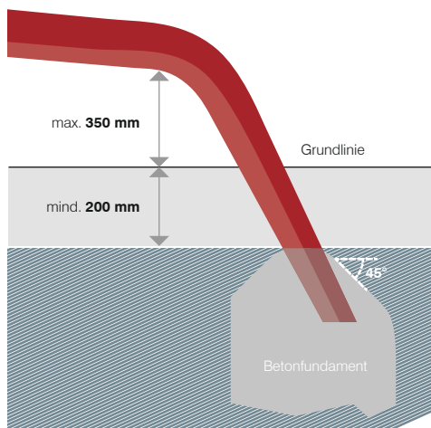
Bild 3 | Ausstiegsteil Betonfundament
