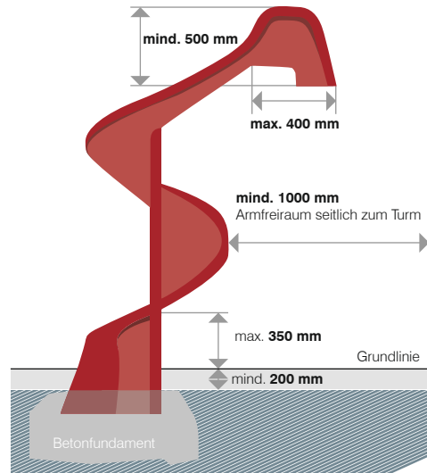
Bild 6 | Wendelrutsche
