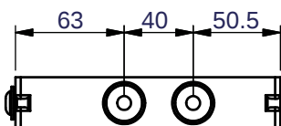
AI[1PCS] 8321-040
