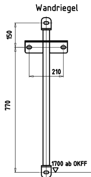
Abb. 5: Bohrungsmaße
