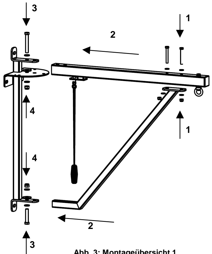
Abb. 3: Montageübersicht 1 (Perspektive)
