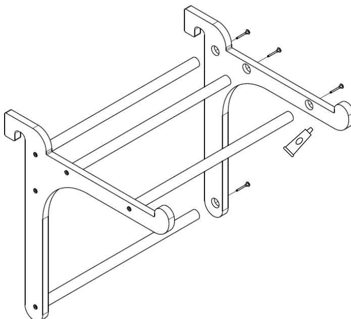
Abbildung 4: Montage rechtes Seitenteil
