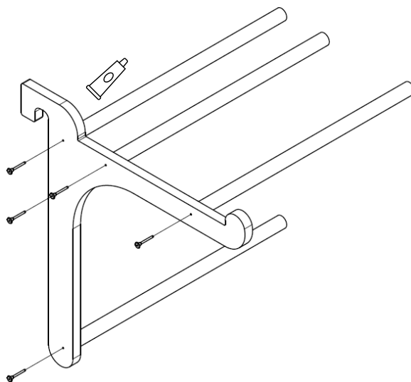
Abbildung 3: Montage linkes Seitenteil
