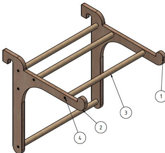
Abbildung 2: Multibügel "Wood"
