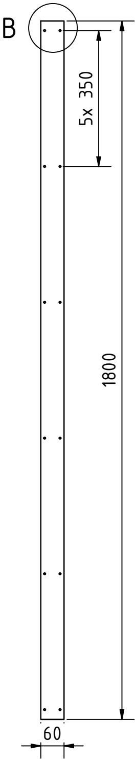
Kunststoffband (2x) ( 1 : 10 )
