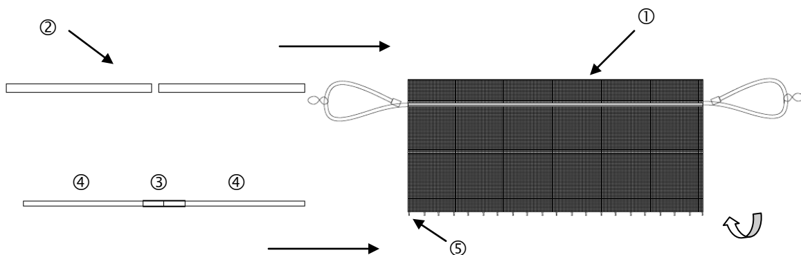
Abbildung 2: Steckverbindung PVC-Stäbe
