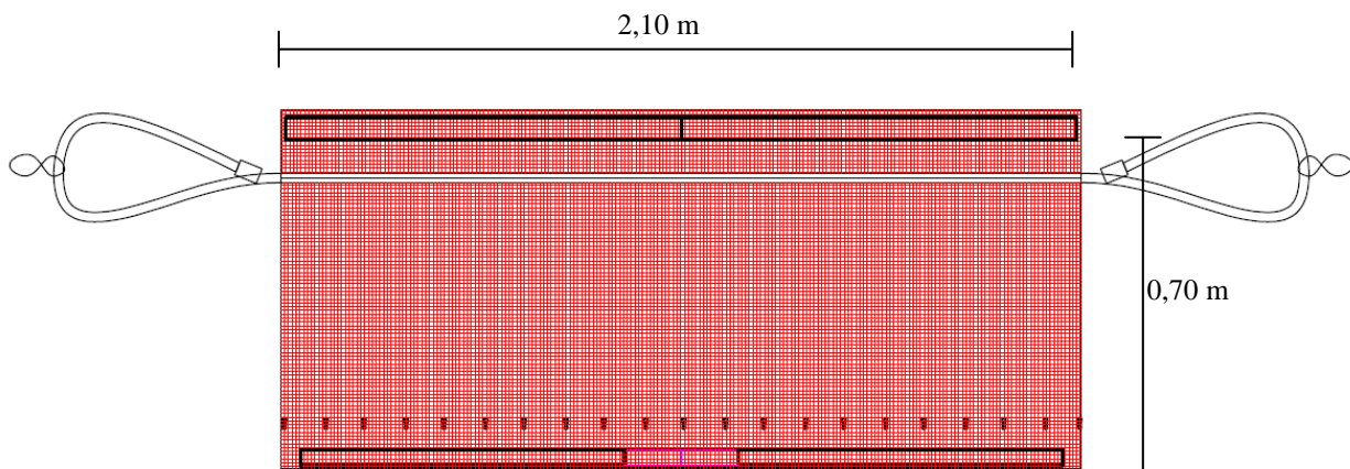
Abbildung 1: Tauchhindernis
